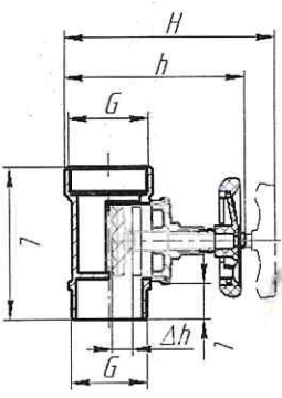
Рисунок 1 – Внешний вид клапанов угловых моделей КТД, КТЧ, КТК и КТММ, КТЧМ, КТКМ
